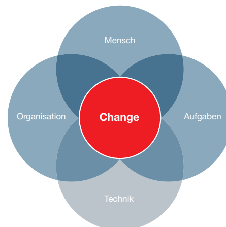
ATOM-Modell
